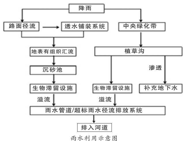
雨水利用示意图
